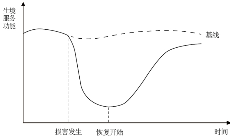
图 B.2 生态环境恢复过程（受损生态环境无法恢复至基线）
